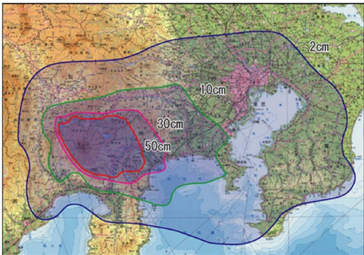
降灰の影響想定範囲
