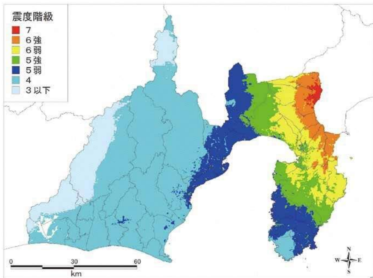
震度分布図（相模トラフレベル1 大正型関東地震）
