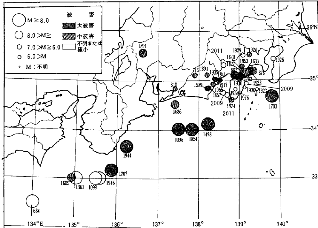
静岡県内の地震活動
