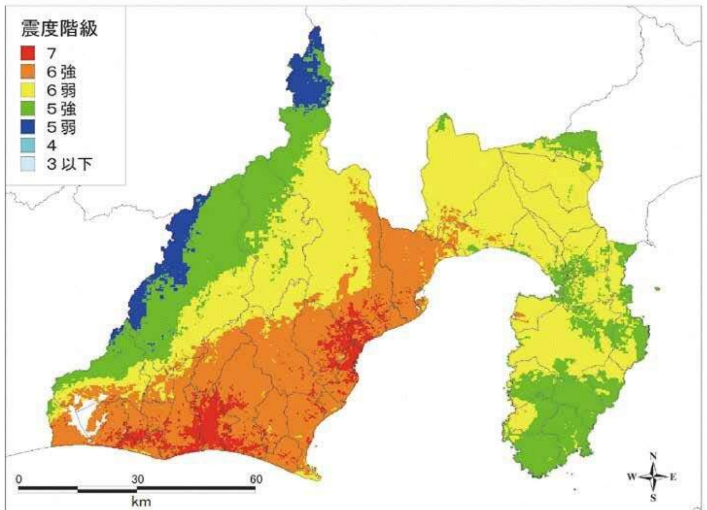
震度分布図（南海トラフレベル1 東海・東南海・南海地震） (注)内閣府(2012)の南海トラフ巨大地震の基本ケースの強震断層モデルを用いて計算したもの
