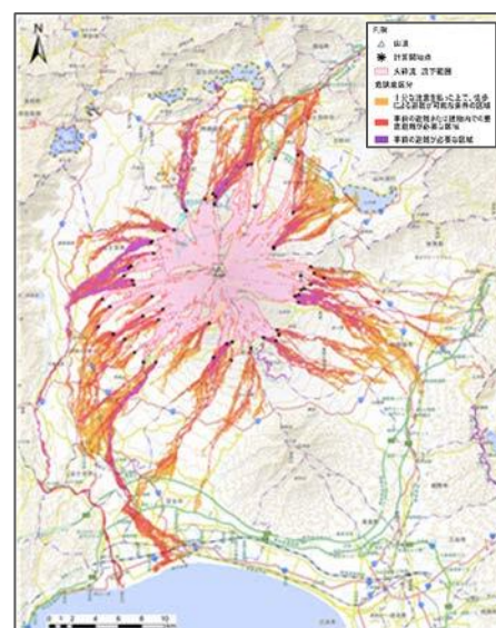
融雪型火山泥流ドリルマップの重ね合わせ図 (危険度区分)
