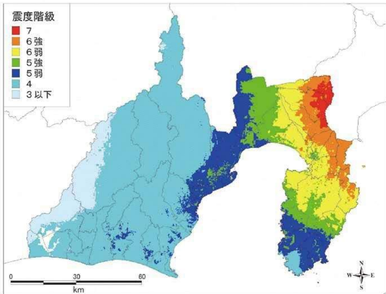
震度分布図（相模トラフレベル2 元禄型関東地震）
