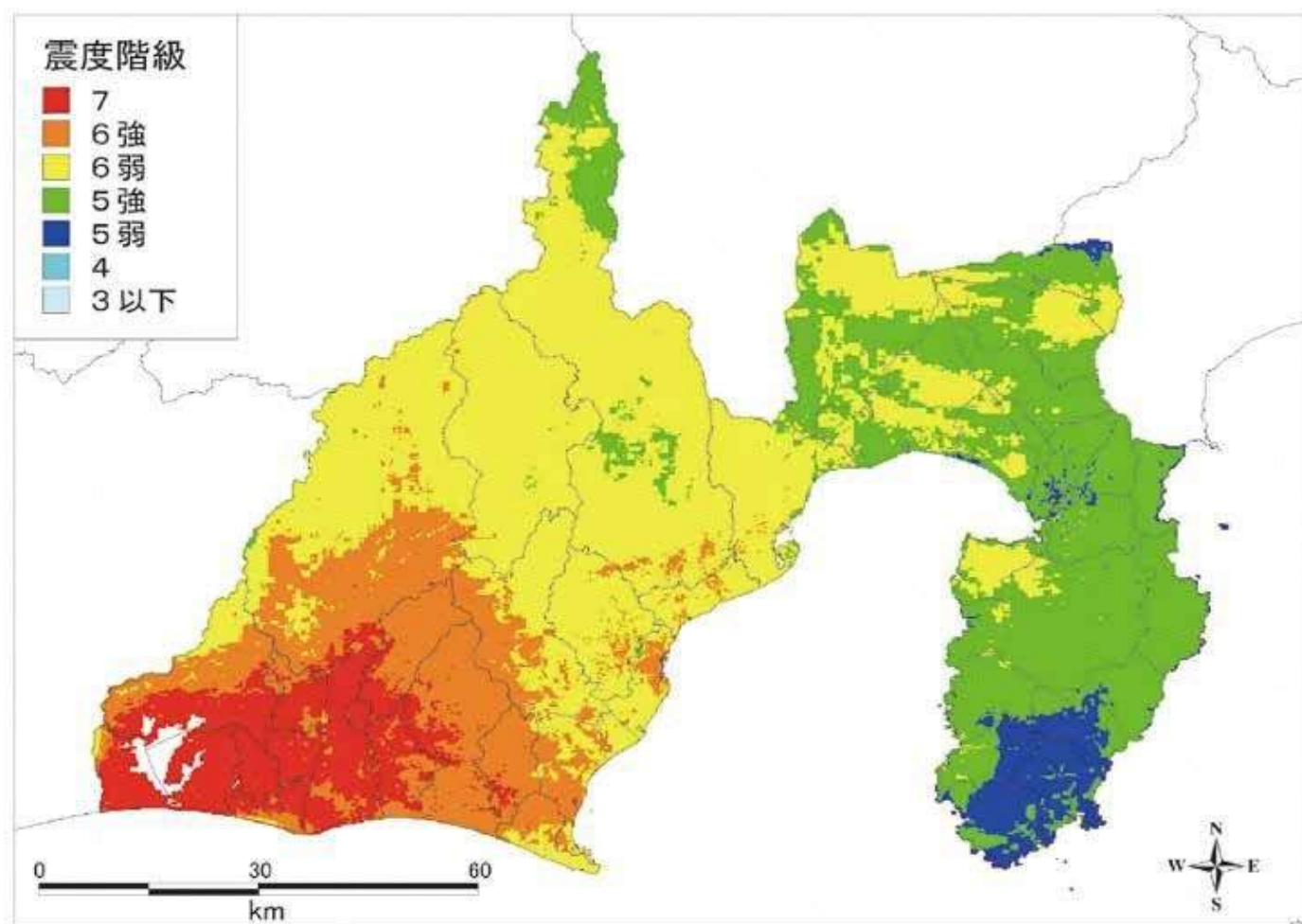
震度分布図 (南海トラフレベル2 南海トラフ巨大地震 陸側ケース)
