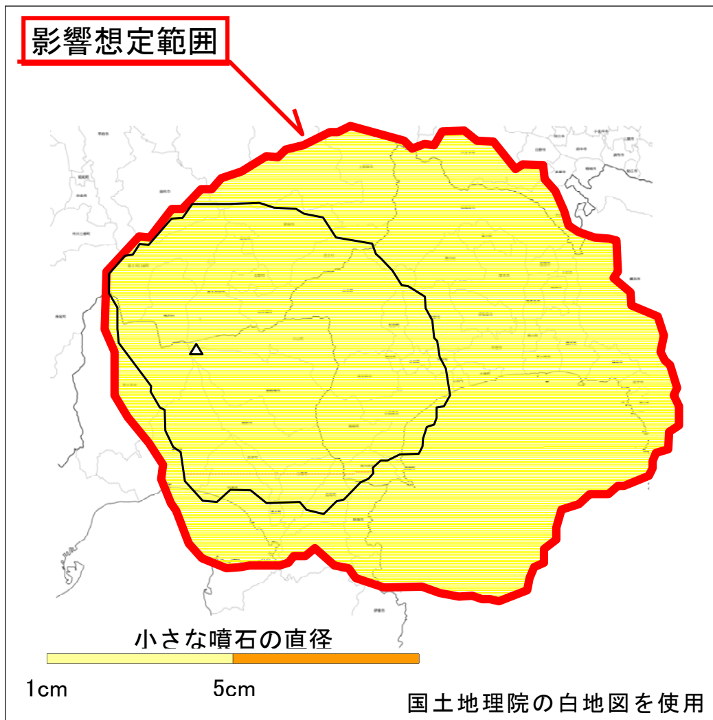
小さな噴石の影響想定範囲
