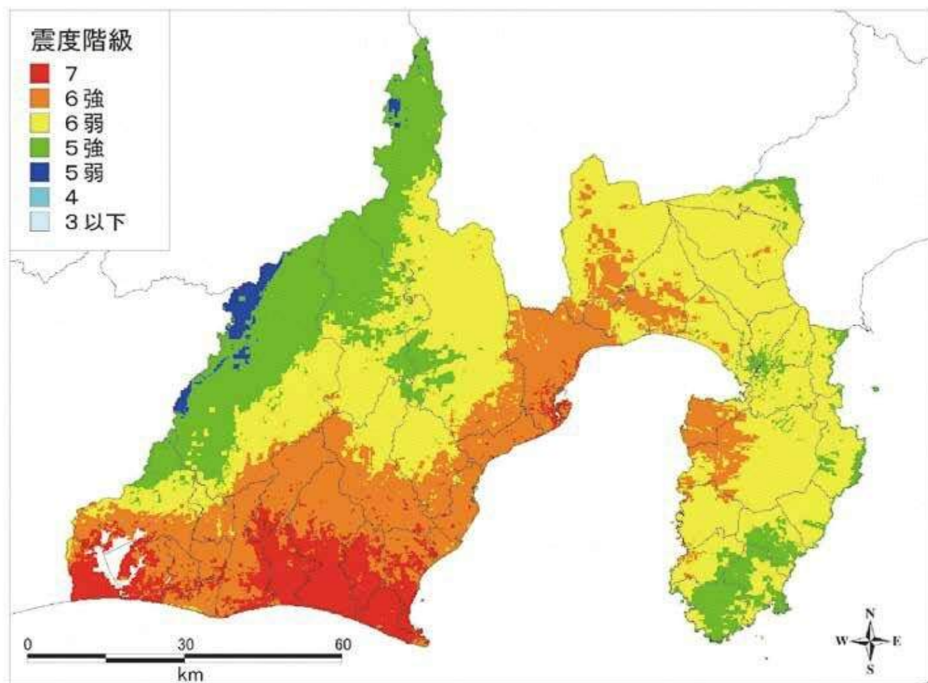
震度分布図（南海トラフレベル2 南海トラフ巨大地震 東側ケース）
