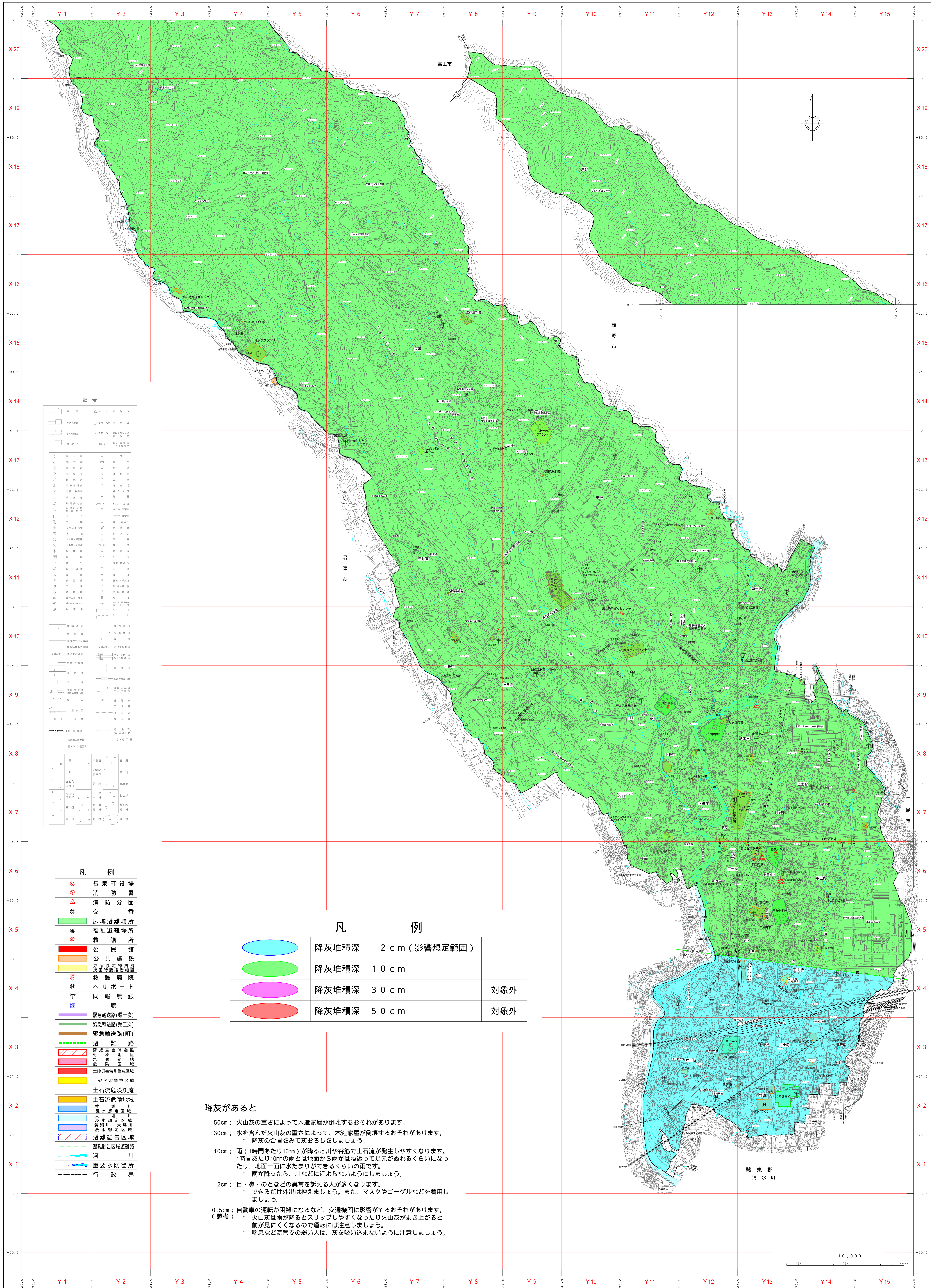
降灰可能性マップ
